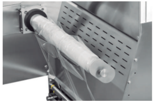
Recogedor automático de film
