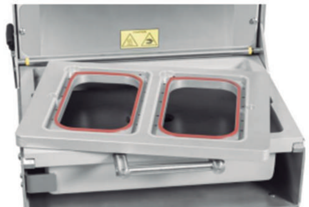
Cambio de moldes rápido / sencillo Medidas máx bandeja 325x265mm
