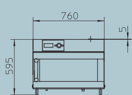
Vista delantera
