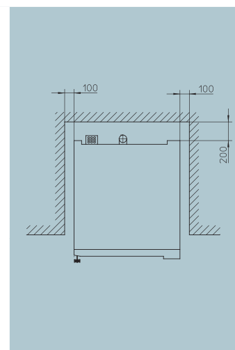
Vista superior
